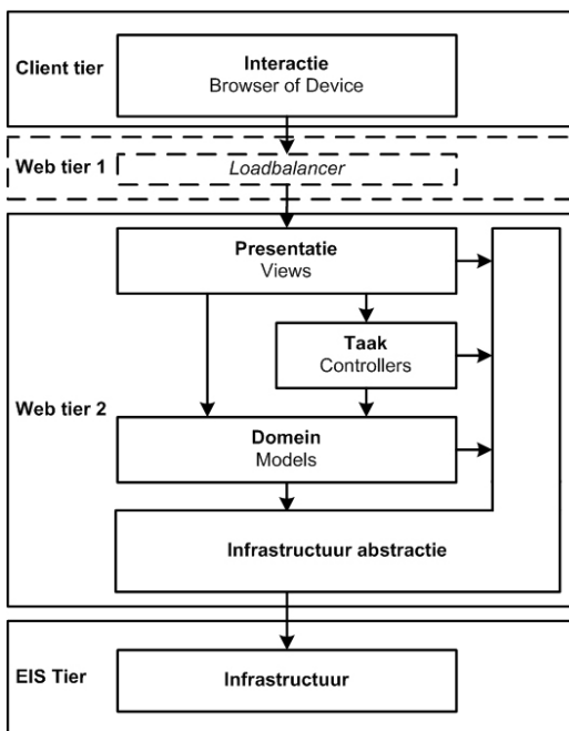
Figuur 4: Het fysieke model op tiers gepositioneerd.
