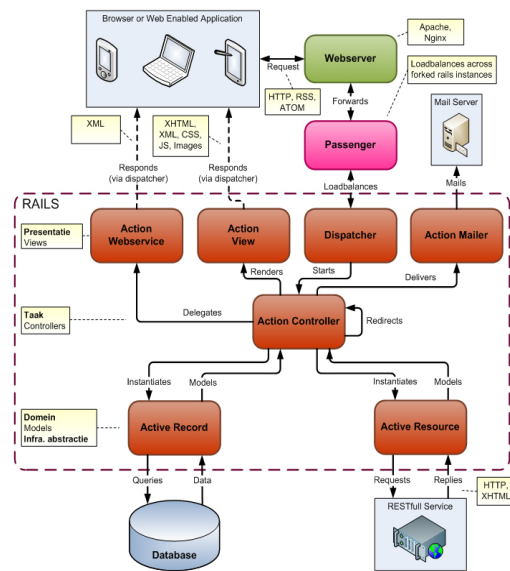
Figuur 2: Ruby on Rails detail fysieke software architectuur.
